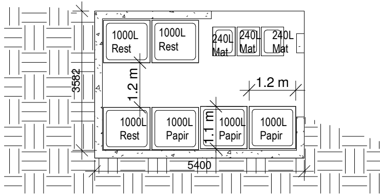
Plan 01 1 : 100
